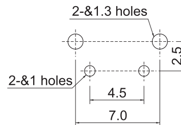
P.C.B.Land Pattern
