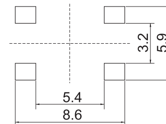
P.C.B.Land Pattern
