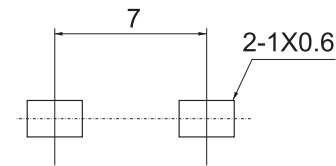
P.C.B.Land Pattern
