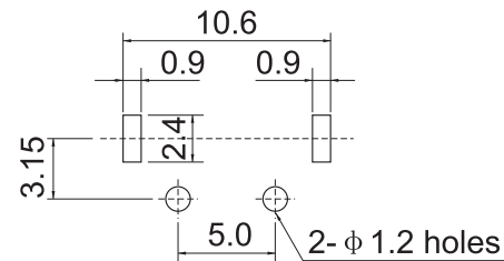
P.C.B.Land Pattern
