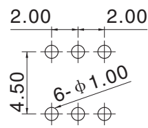
PCB Layout(Pattern Side)
