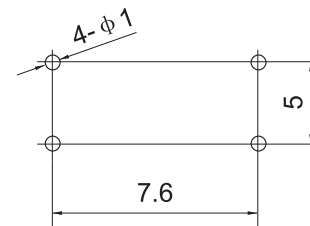
P.C.B.Land Pattern
