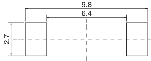
P.C.B. Land Pattern
